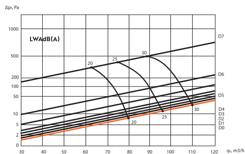
LINEO PRO 20 mm slot (odvod vzduchu)
