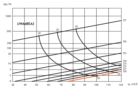
LINEO PRO 20 mm slot (přívod vzduchu)
